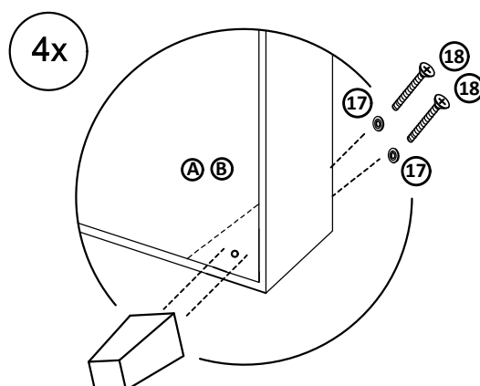
Montáž nôh typu GRN:
