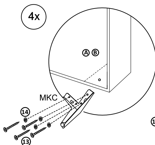
Montáž nôh typu MKC:
