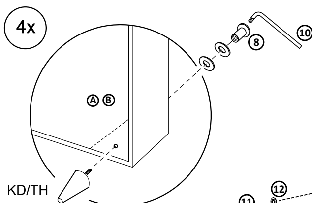
Montáž nôh typu KD:
