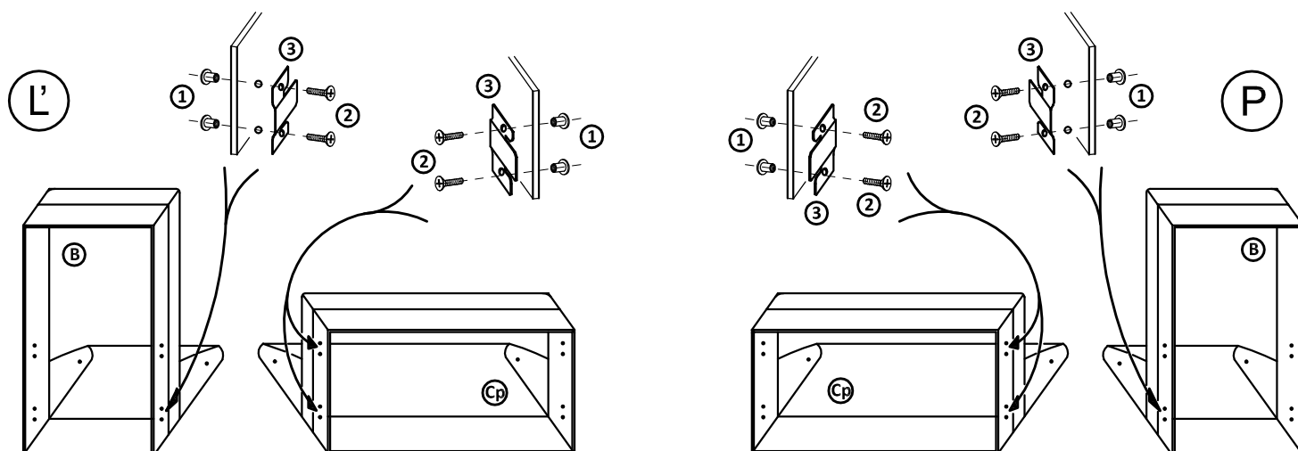
Montáž spojovacieho háku na prístavok a dvoj kreslo pevné
