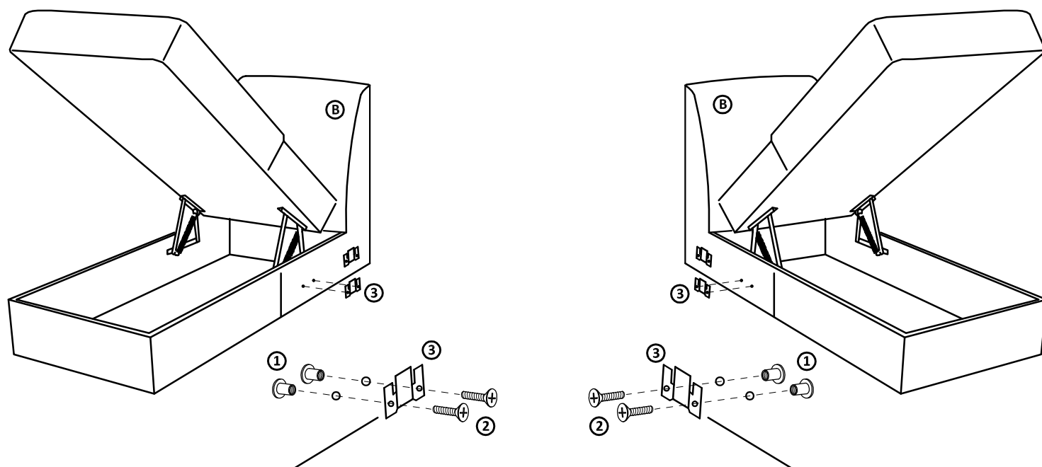
Montáž spojovacieho háku na prístavok z úložného priestoru
