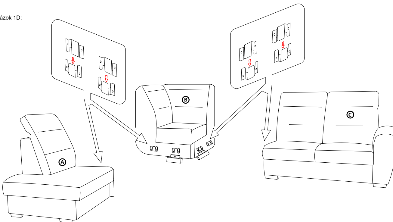
Elementy spojte zaháknutím spojovacieho háku
