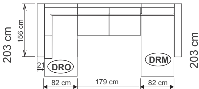
súprava DU-3SR160-DRO :
