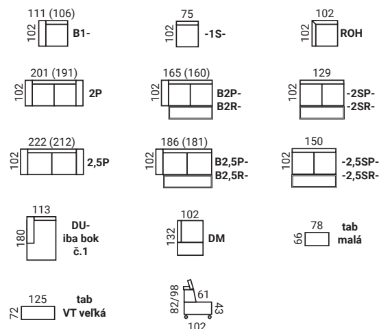
B2P-B (bok č. 2 pevné)
